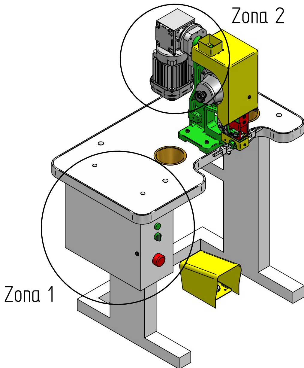
Figura 1 – Zonas de Risco Elétrico da Máquina Rebitadeira MR11
